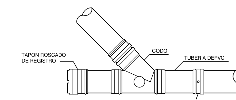
DETALLE REGISTRO COLECTORES - (PLANTA)
