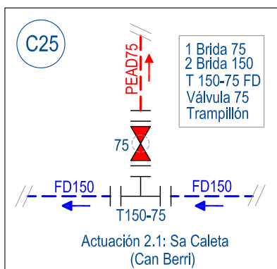
Esquema Conexiones: Sin Escala
